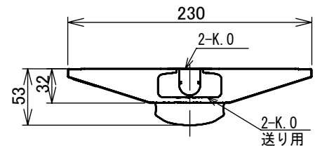
側面詳細図
