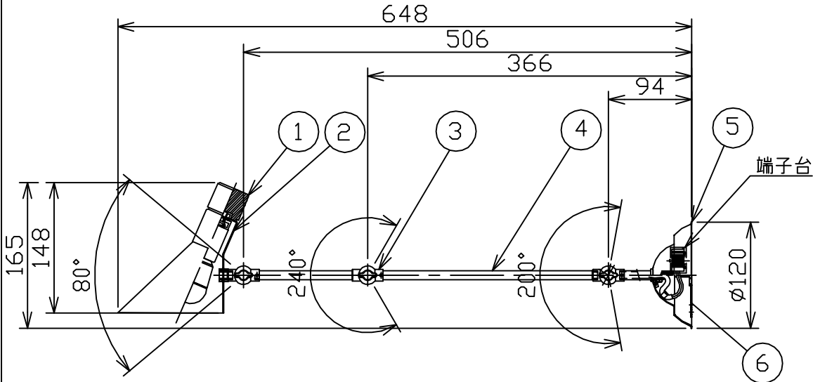
取付部詳細
