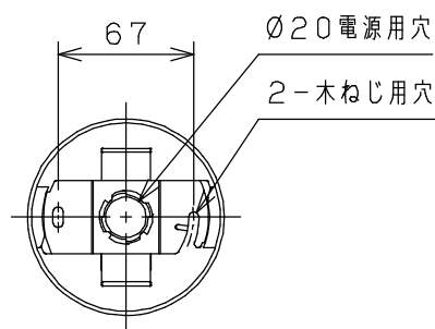
取付部詳細
