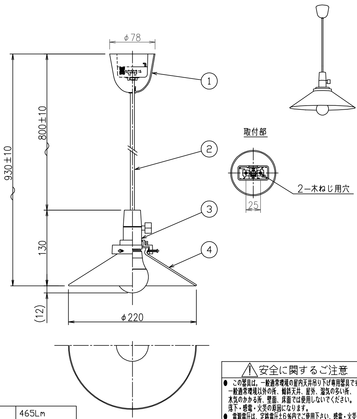
姿図
