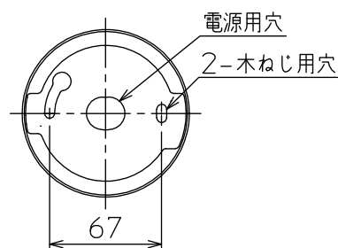
取付部詳細
