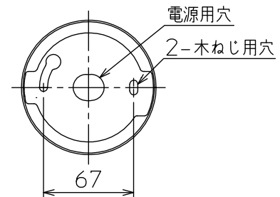
取付部詳細
