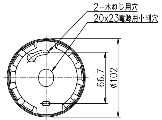
取付詳細図
