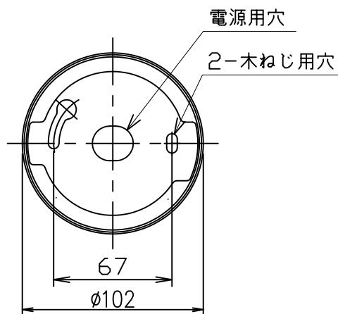
取付部詳細
