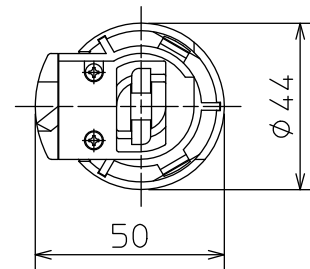
取付部詳細
