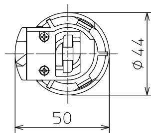
取付部詳細
