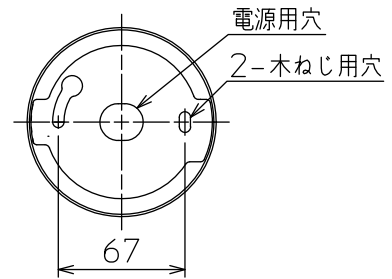
取付部詳細
