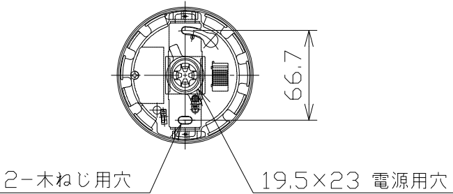
取付部詳細
