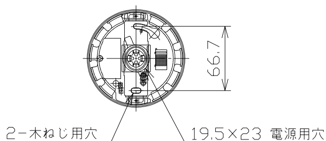
取付部詳細
