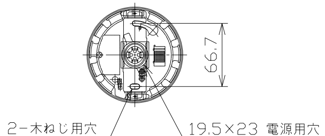
取付部詳細
