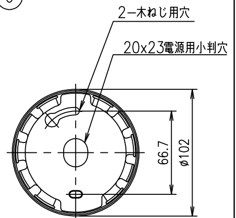
取付詳細図
