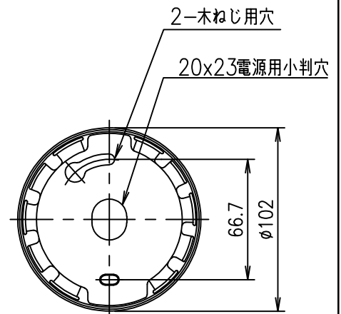
取付詳細図
