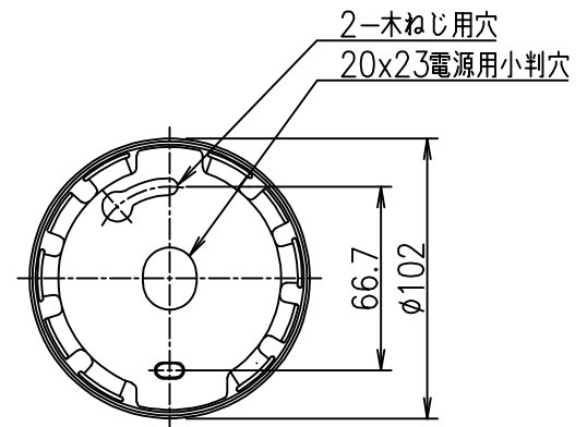
取付詳細図
