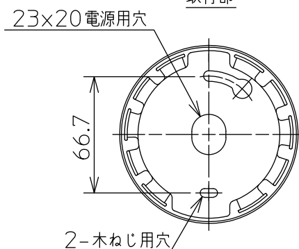
取付部
