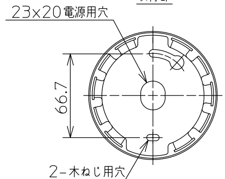
取付部
