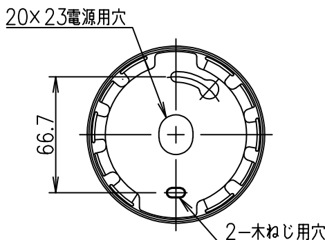
取付部詳細
