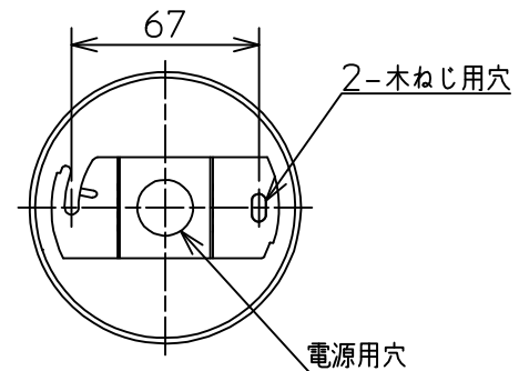
取付部詳細
