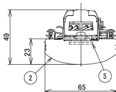
側面詳細図
