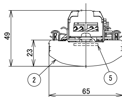
側面詳細図
