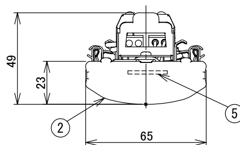
側面詳細図
