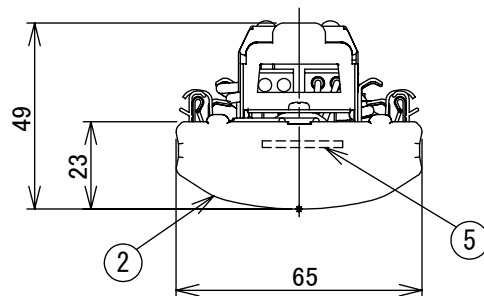
側面詳細図
