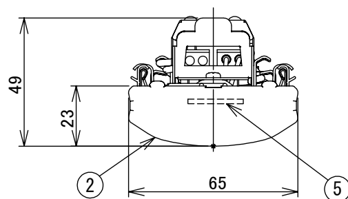
側面詳細図
