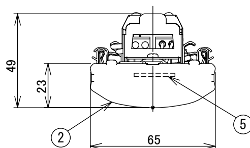
側面詳細図
