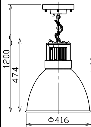
セード組合せ時寸法 (乳白カバー・透明カバー・アルミカバー大)
