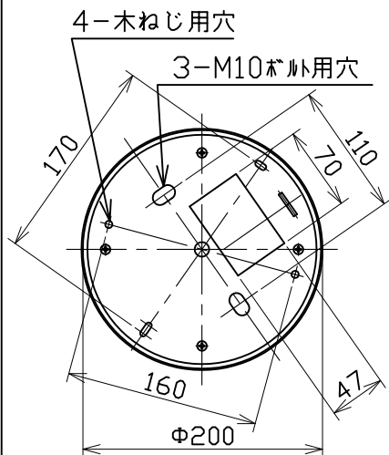
取付部詳細
