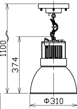
セード組合せ時寸法 (アルミカバー小)
