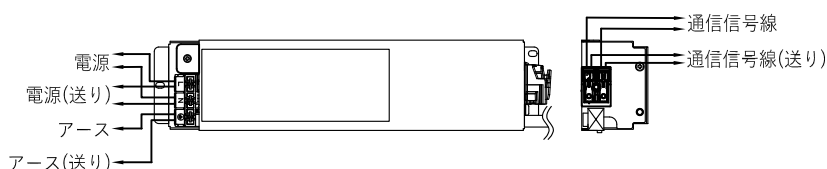
結線図
