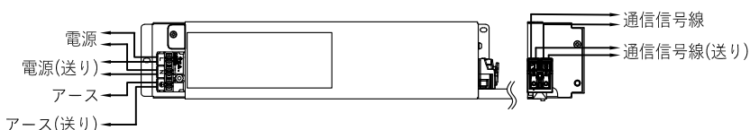
結線図
