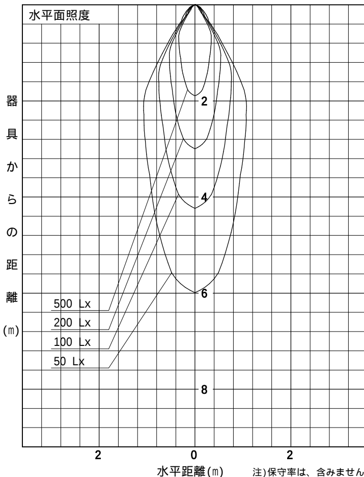
配光曲線
