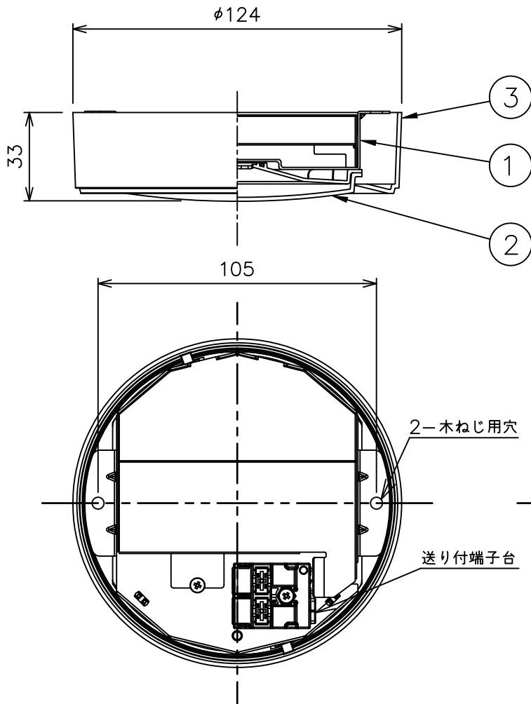
取付部詳細
