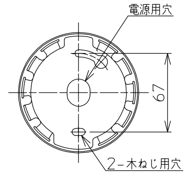
取付部詳細
