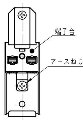
端子台詳細
