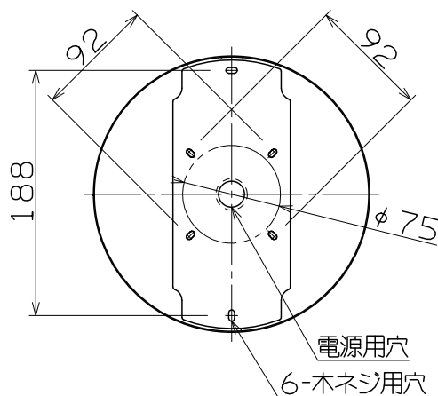
取付詳細図
