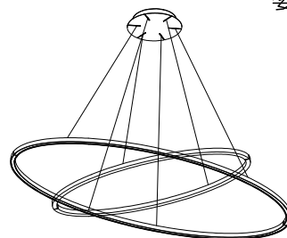
姿図
