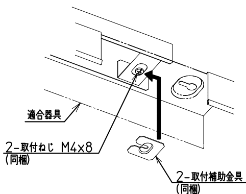
A 矢視図 器具取付部
