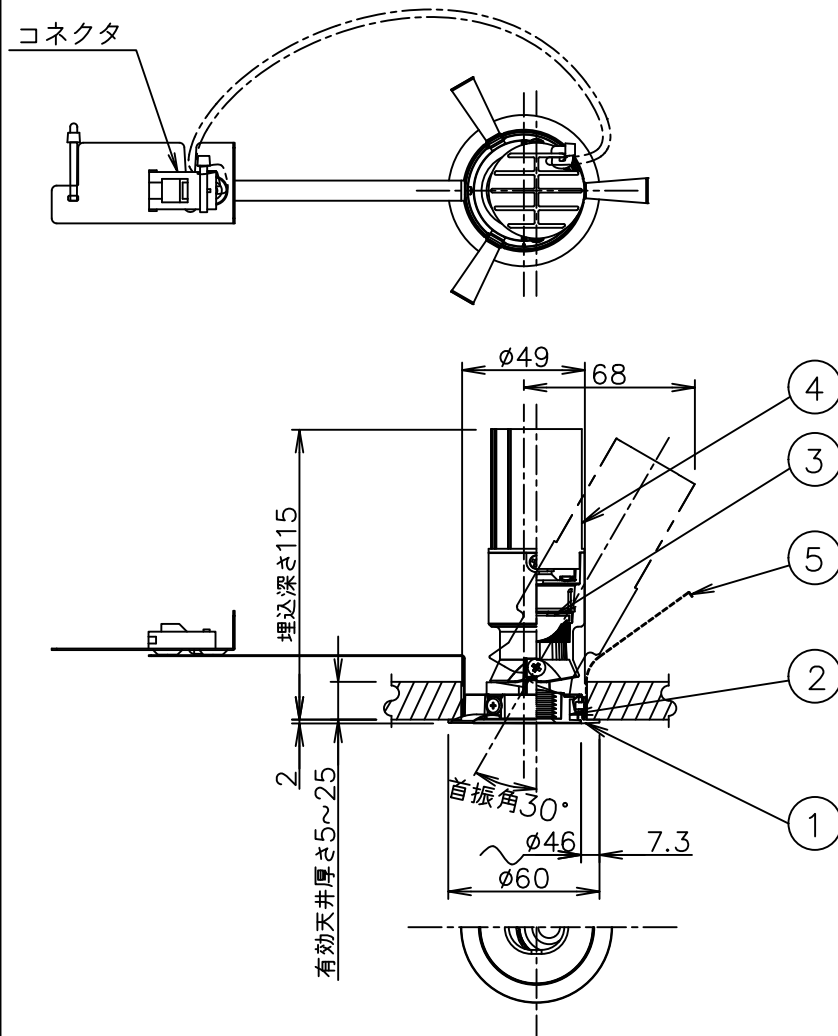
埋込穴寸法
