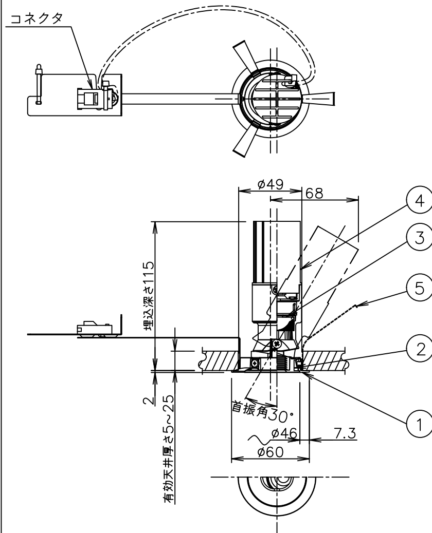
埋込穴寸法
