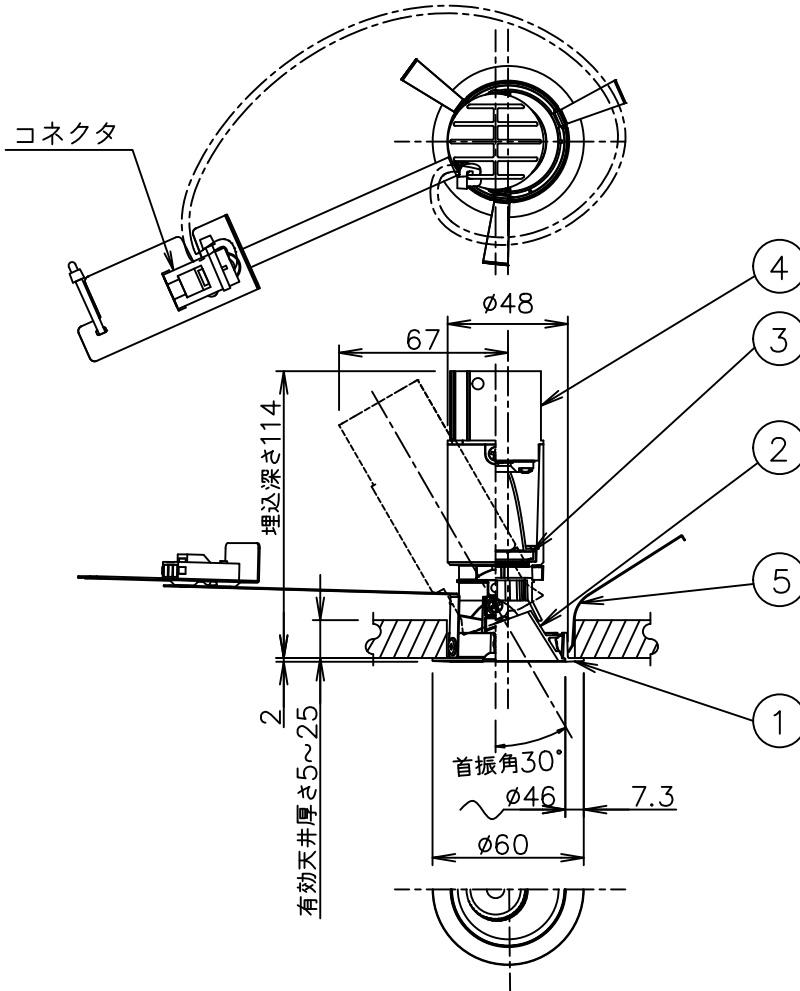
埋込穴寸法
