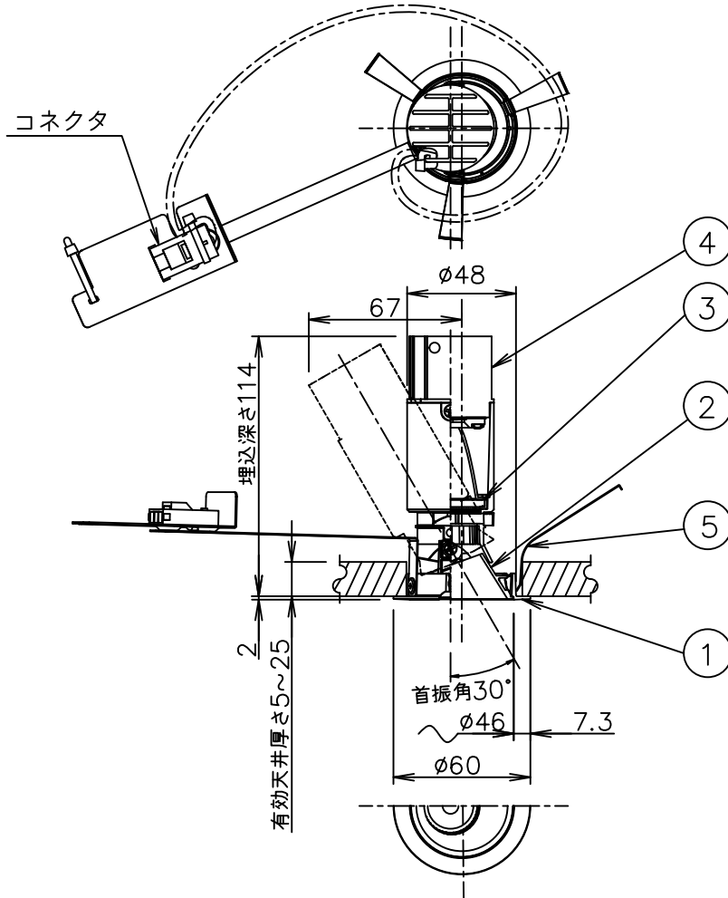
埋込穴寸法
