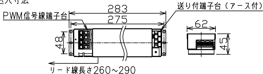
埋込穴寸法
