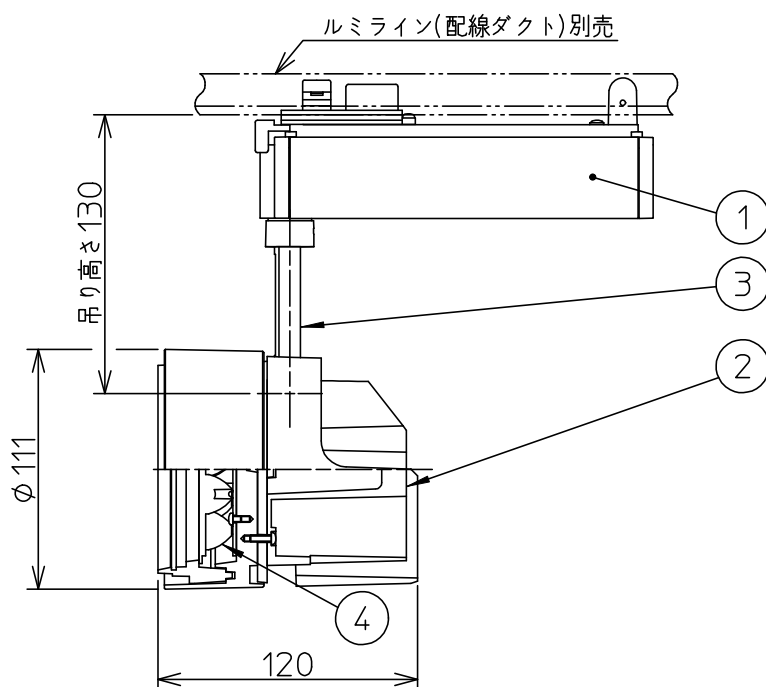
取付部
