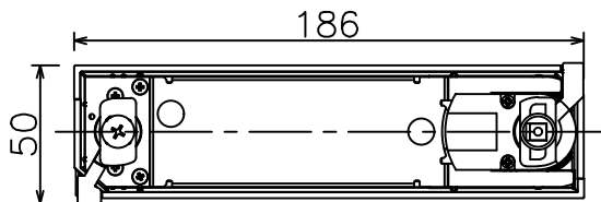
取付部
