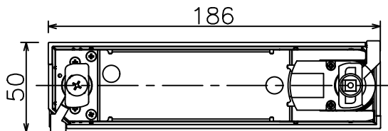
取付部
