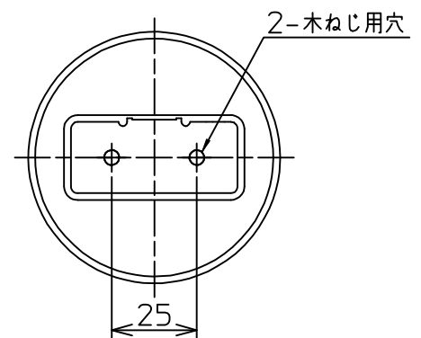
取付部詳細
