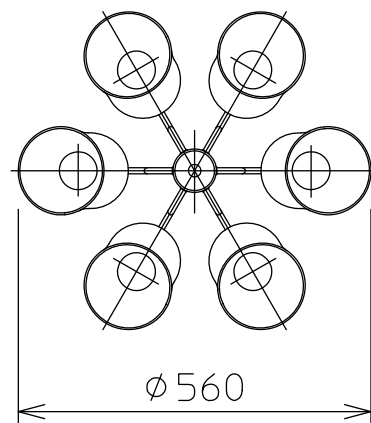
灯具配置図
