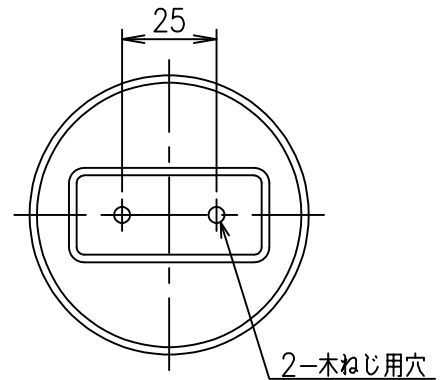
取付部詳細
