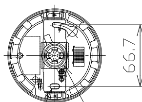
取付部詳細
