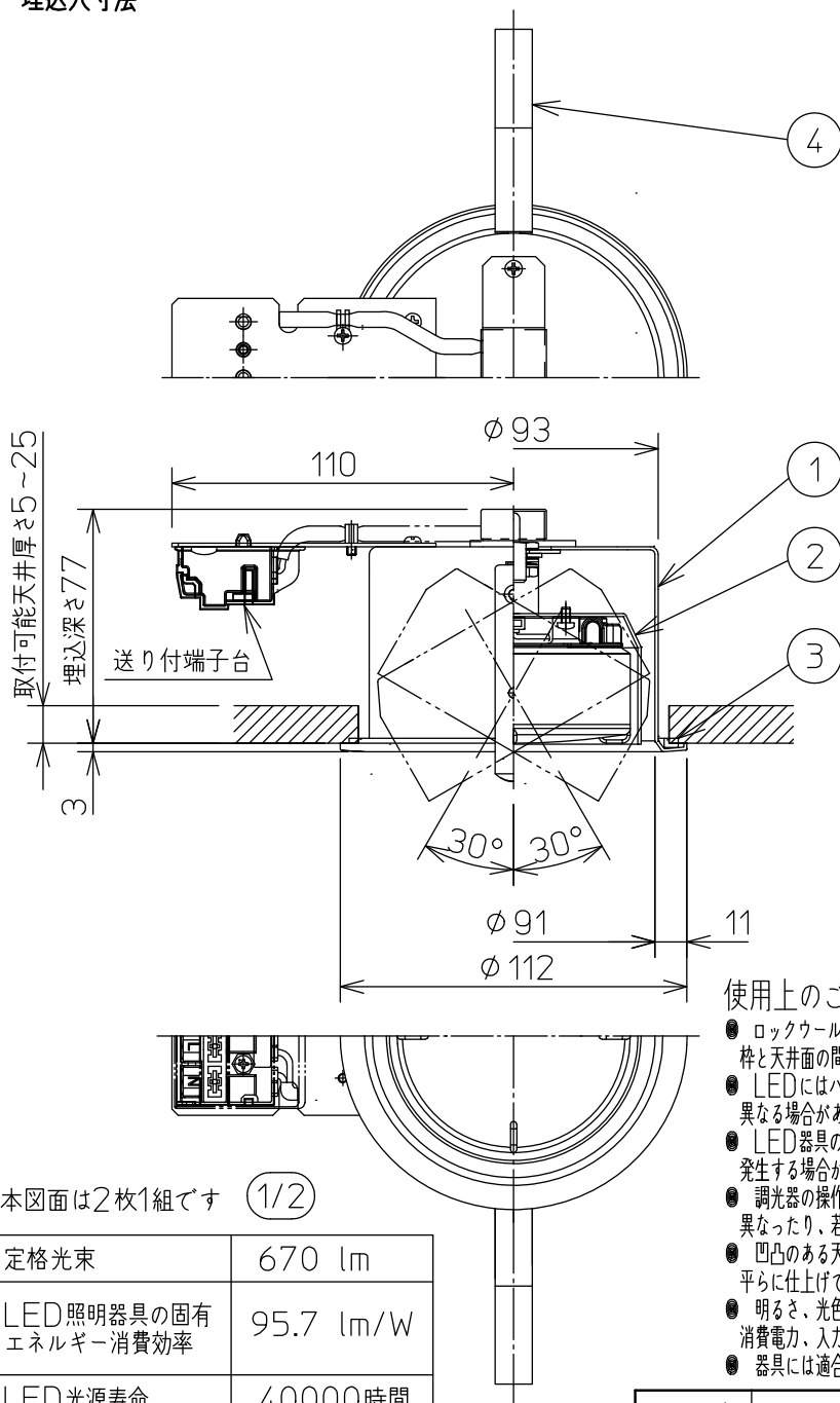
埋込穴寸法
