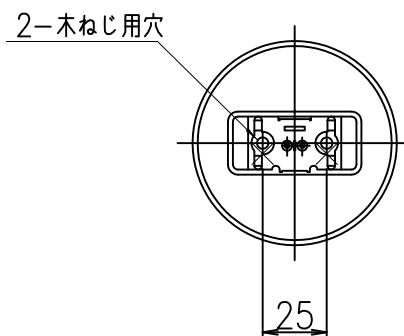
取付部詳細
